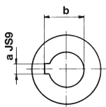
Provedení s drážkou DIN 6885 Příklad pro objednání: 03H-N
