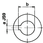
Provedení s drážkou DIN 6885
